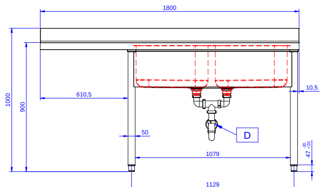
Oldalnézet
